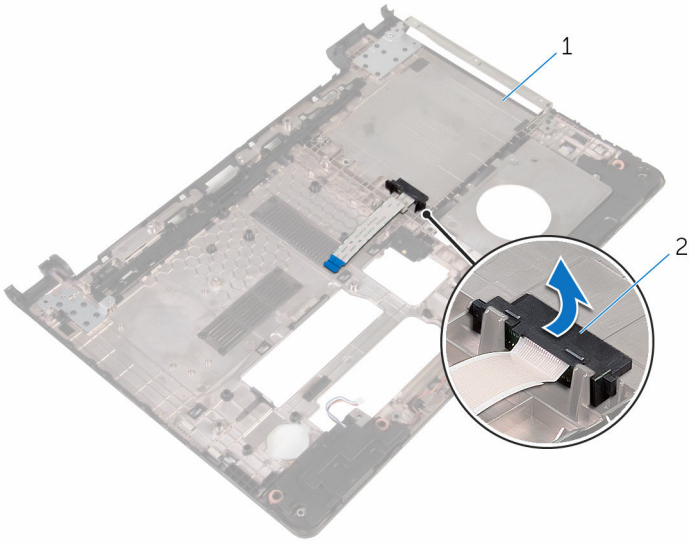
1 Interposer des optischen Laufwerks
